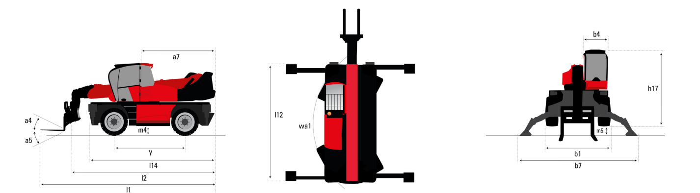
MRT 2145 115 - Diagrama dimensional
